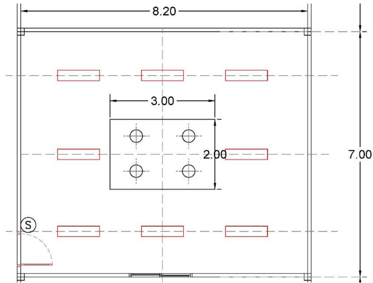
ภาพที่ 1-6 แบบแปลนระบบไฟฟ้า
